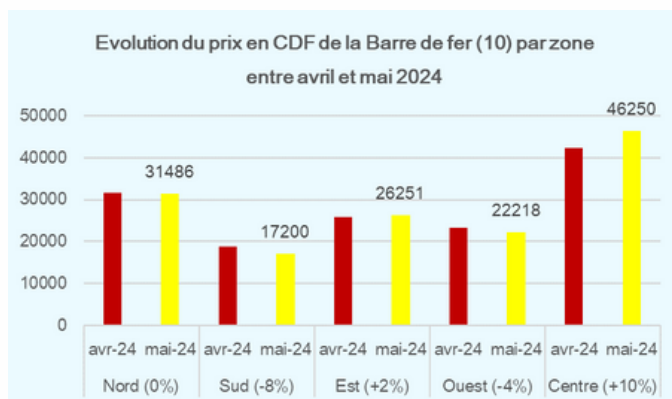
Figure 14 : Prix de bar de fer (10)
