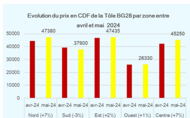
Figure n° 9 : Prix de la tôle (BG 28)
